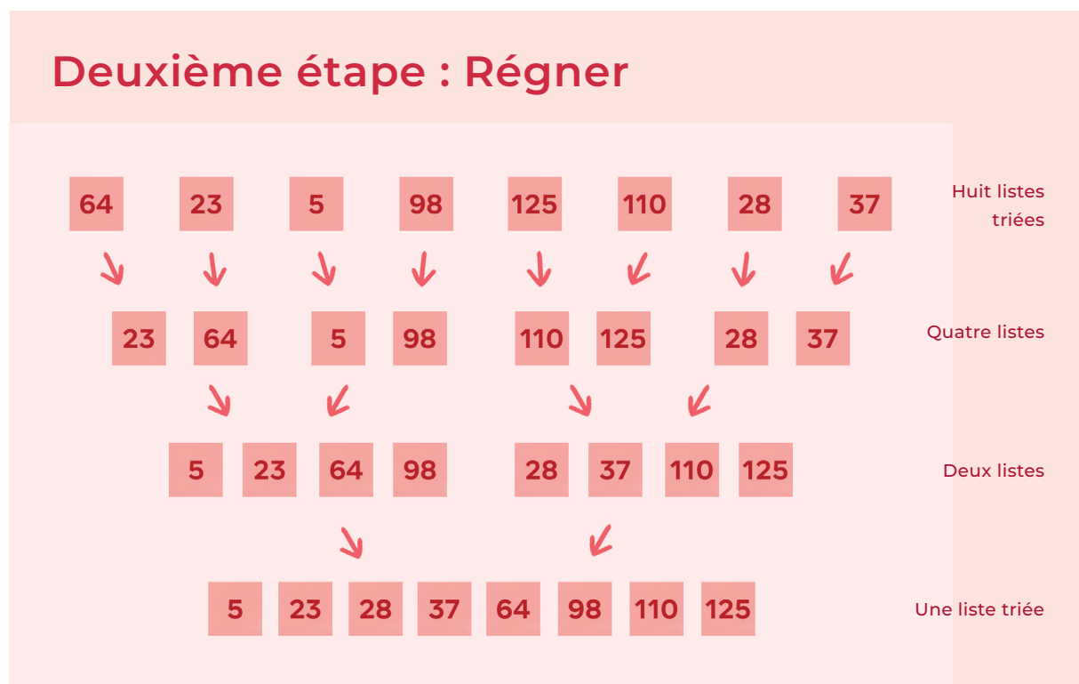
Diagramme de tri fusion - Deuxième étape : Régner
