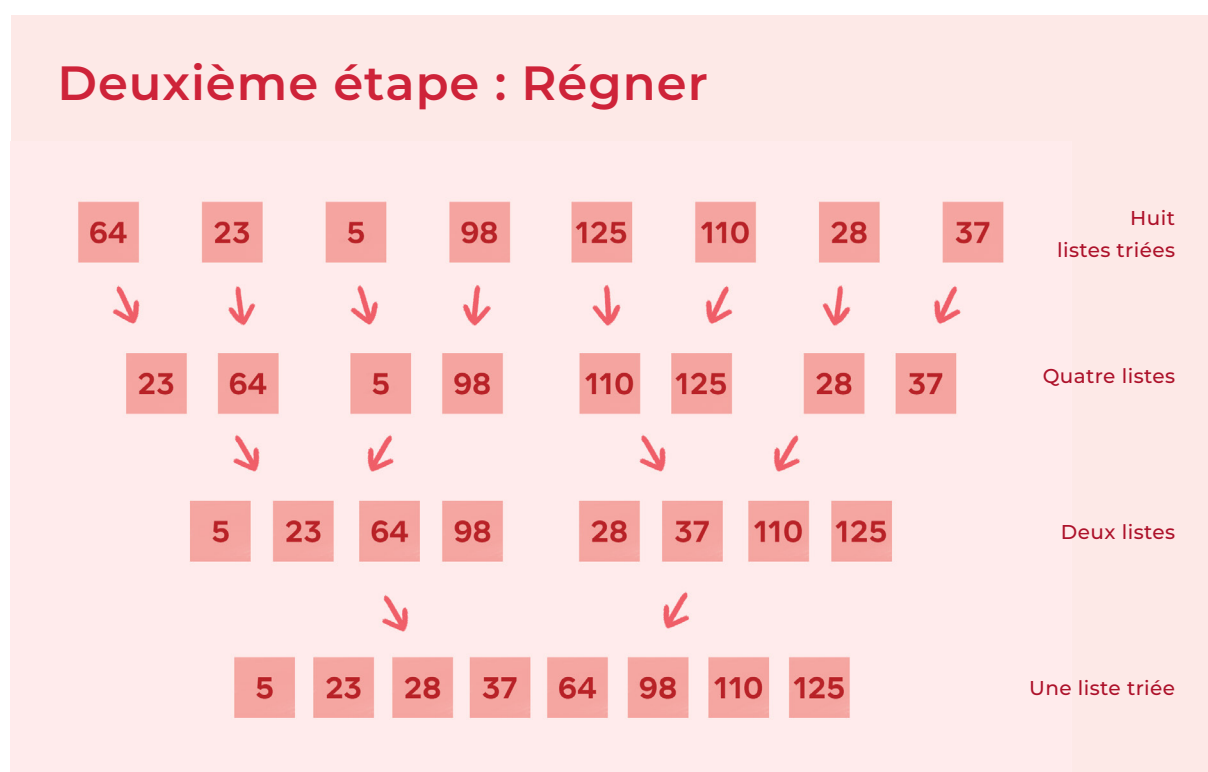
Diagramme de tri fusion - Deuxième étape : Conquérir
